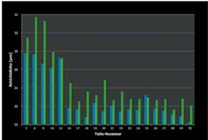
airmatic : Épaisseurs de couches sur des substrats différents
